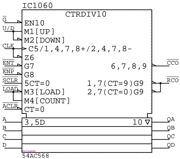
54AC568
