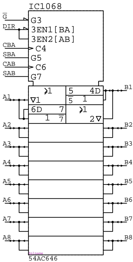
54AC646
