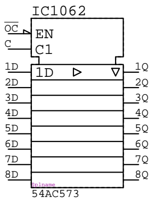
54AC573
