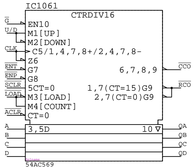
54AC569
