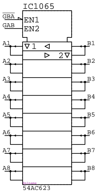
54AC623
