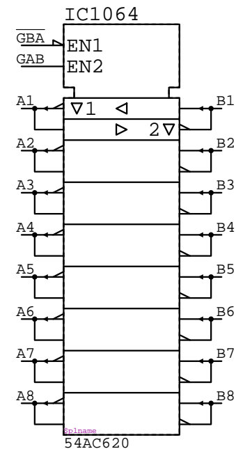
54AC620
