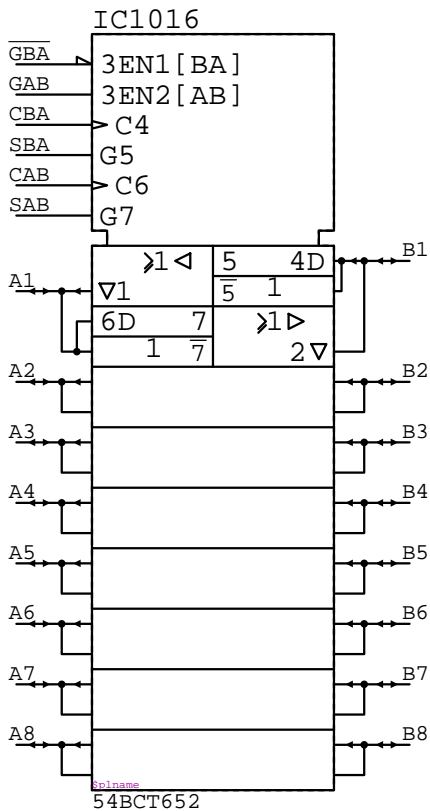
54BCT652
