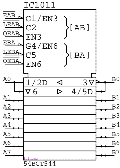
54BCT544
