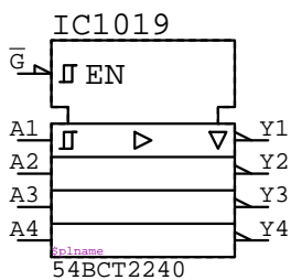
54BCT2240
