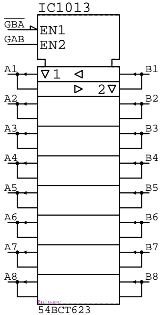
54BCT623
