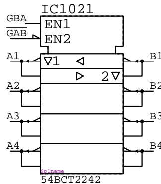
54BCT2242
