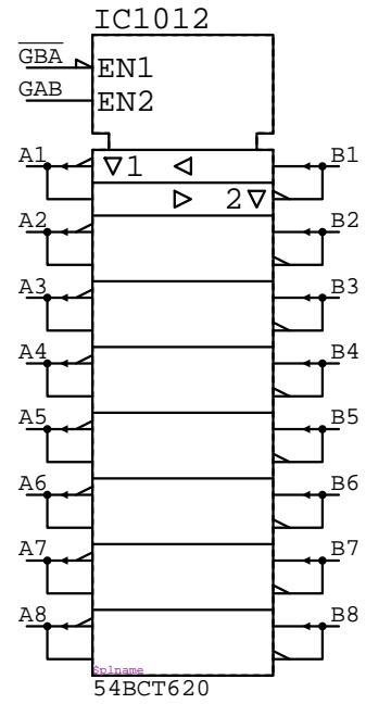
54BCT620
