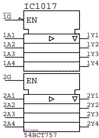
54BCT757
