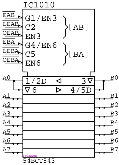
54BCT543
