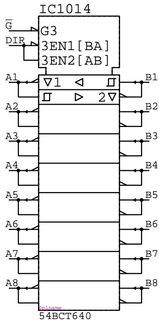
54BCT640
