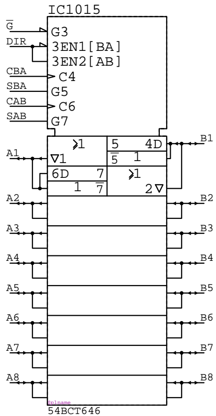
54BCT646
