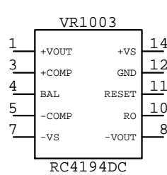
VR_RC4194D VR?????
