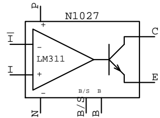
OP_LM311 N????
