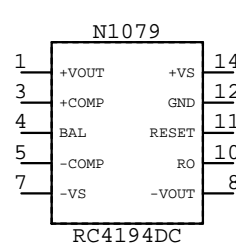
VR_RC4194DC N?????
