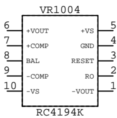
VR_RC4194K VR?????
